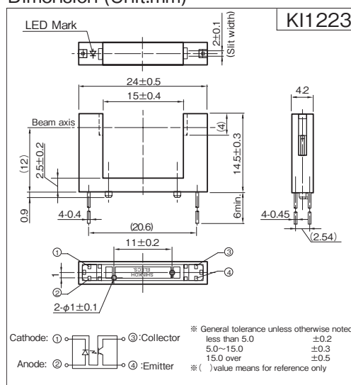
Dimension (Unit:mm)
